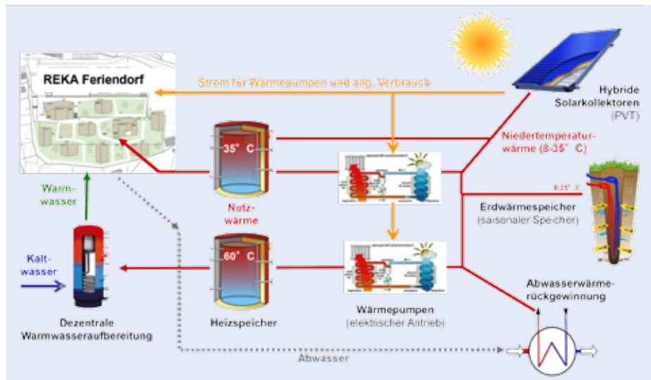
Das Energiesystem des Feriedorfs Blatten-Belalp im Überblick. (Bild: Elimes AG)
