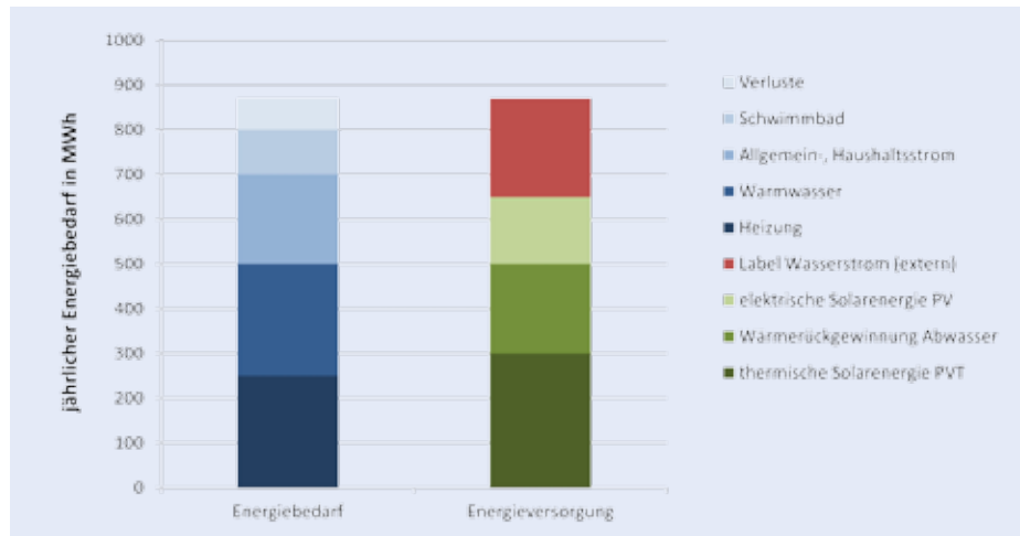
Die (rechnerische) Energiebilanz des Reka-Feriedorfs in Blatten: Auffällig ist bei den Verbräuchen (links) der relativ hohe Anteil für Warmwasser, wie er typisch ist für einen Hotelbetrieb. Rechts: Gut die Hälfte der Energie kommt direkt von der Sonne, weitere 20 % werden von der Anlage zur Abwasserwärmerückgewinnung gedeckt. Hinzu kommen 30 % Strom aus dem Netz (zertifizierter Ökostrom aus Wasserkraft). Die Verluste liegen bei 10 %, was für ein Arealnetz mit Rohrleitungen üblich ist. (Bild: Lauber Iwisa AG)
